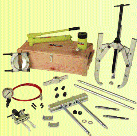
Estrattore a griffe
